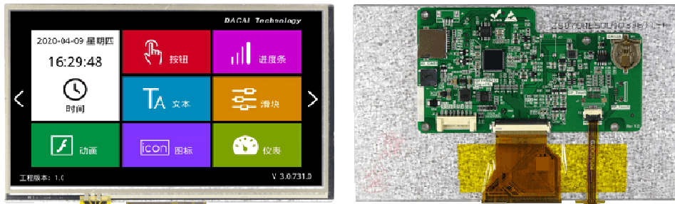
图 1-1 7.0 寸电阻触摸参考图
