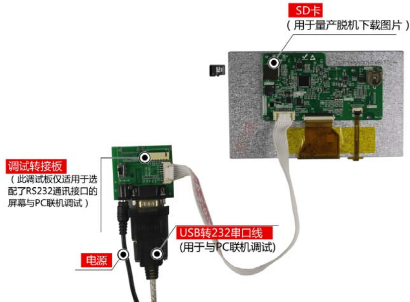
图 1-4 调试工具图
