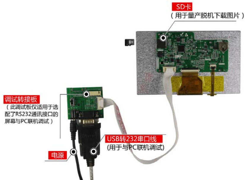
图 1-4 调试工具图
