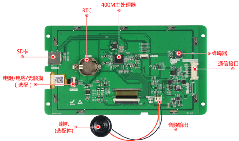
图 1-4 硬件配置图
