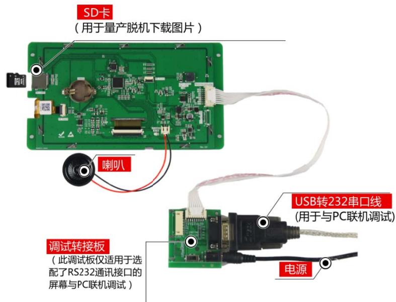
图 1-5 调试工具图
