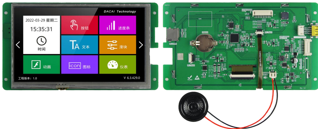
图 1-1 7.0 寸电阻触摸参考图
