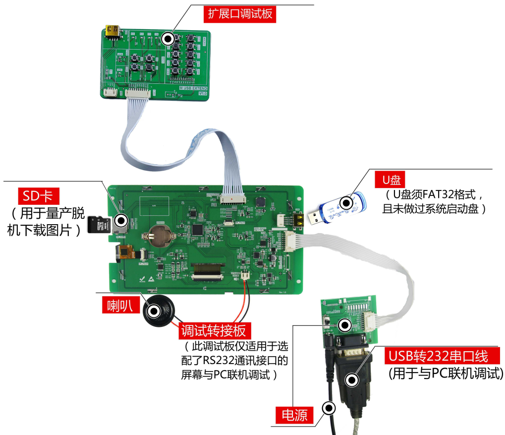
图 1-5RS232 调试工具图
