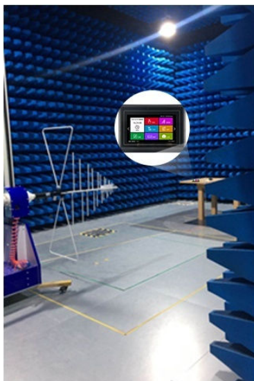
图 6-5 辐射测试图
