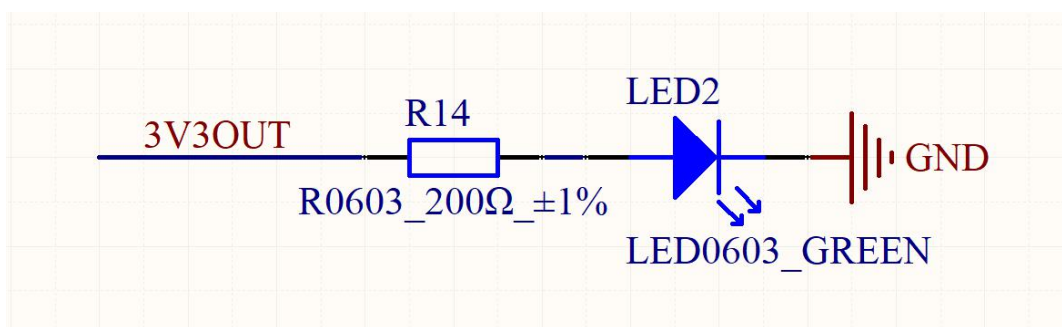
图 16-4 3.3V 为 LED 供电
