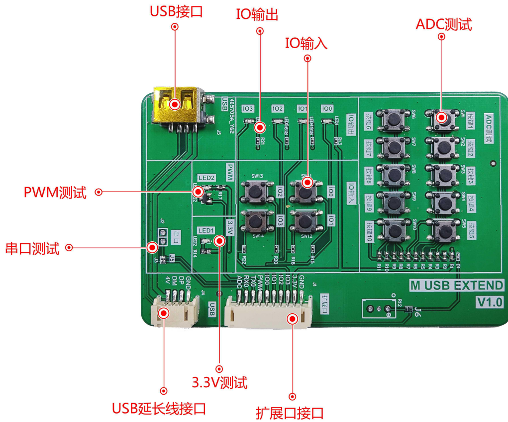
图 5-1 扩展口测试板
