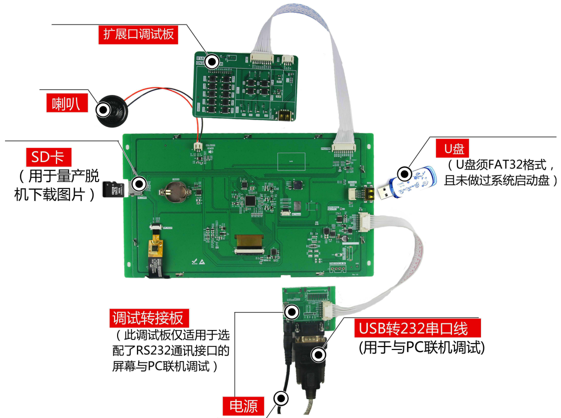
图 1-5 调试工具图
