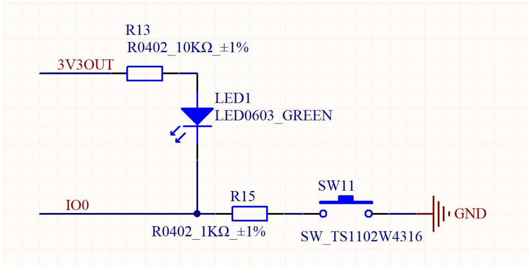
图 16-6 IO 输入、输出
