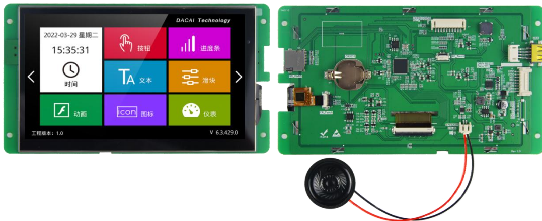
图 16-1 M 系列 7 寸串口屏
