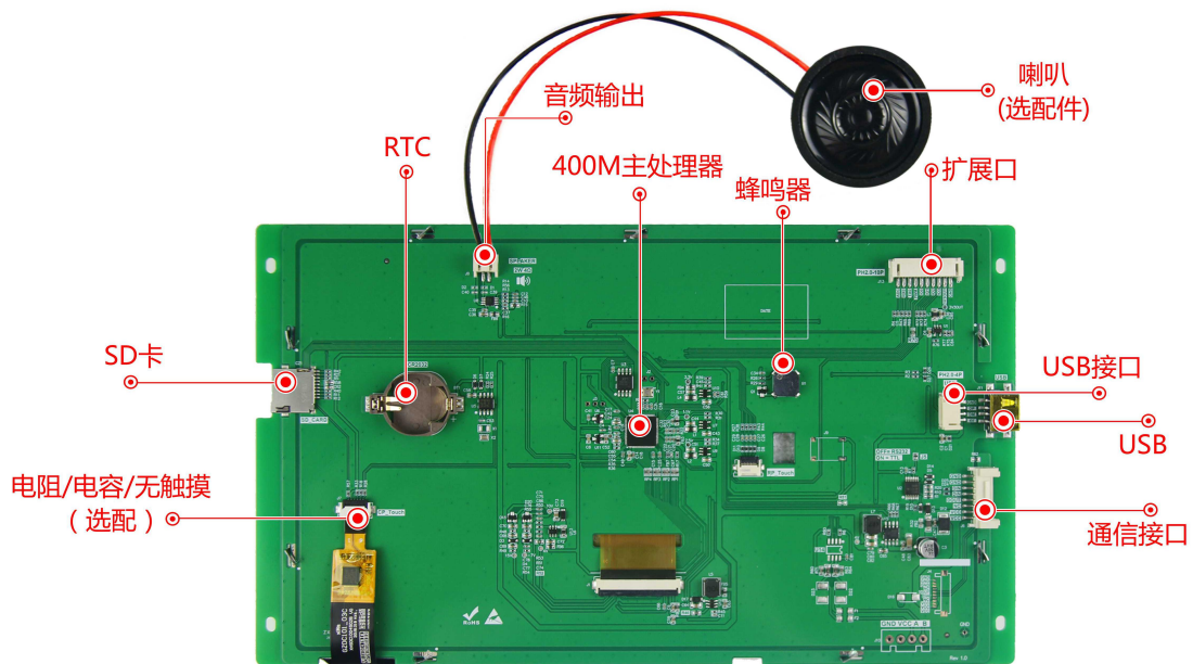
图 1-4 硬件配置图
