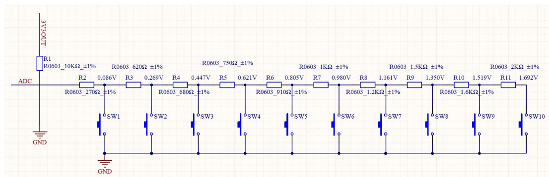
图 16-5 ADC 按键输入
