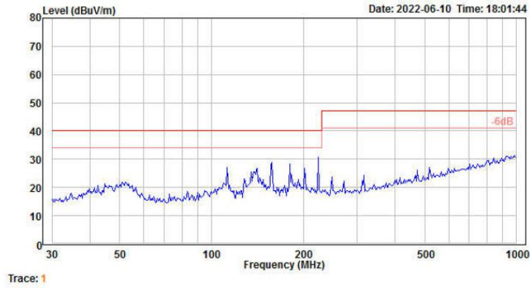
图 6-6 辐射测试水平方向
