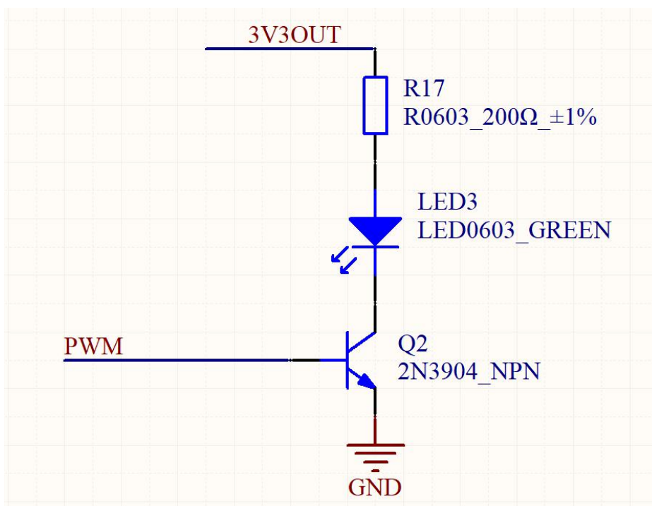
图 16-7 PWM 控制 LED 亮度
